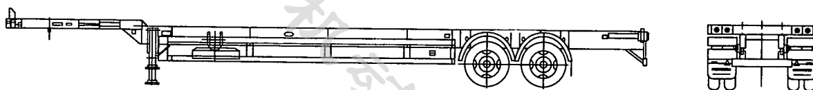
图 A.7 骨架式集装箱运输半挂车
