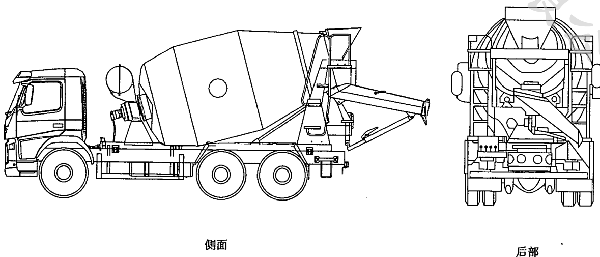
图 A.9 混凝土搅拌运输车
